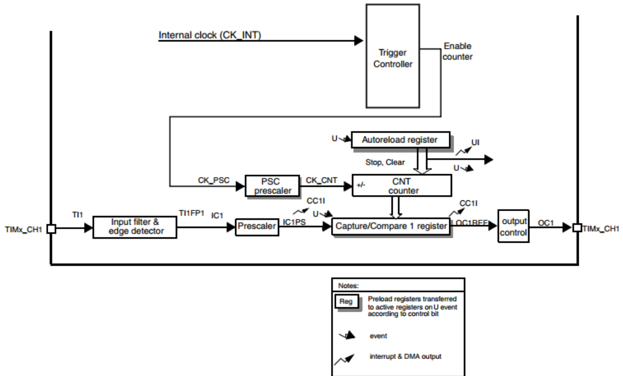
图 16-1 TIMx(TIM10/TIM11/TIM13/TIM14)模块
