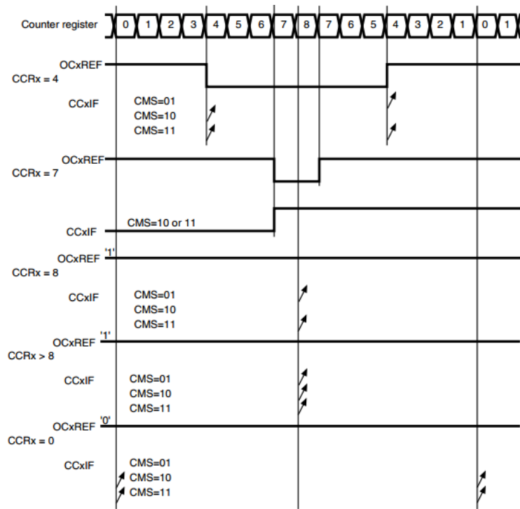
图 14-32 央对齐的 PWM 波形(APR=8)
