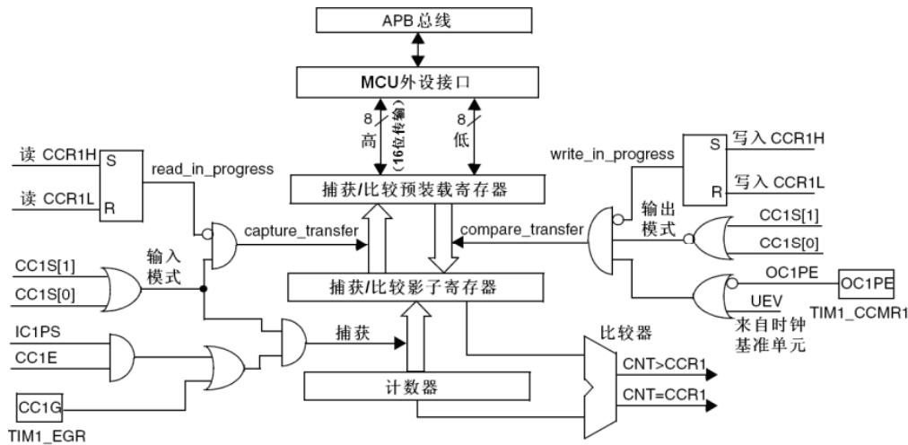
图 14-27 捕获/比较通道 1 的主电路
