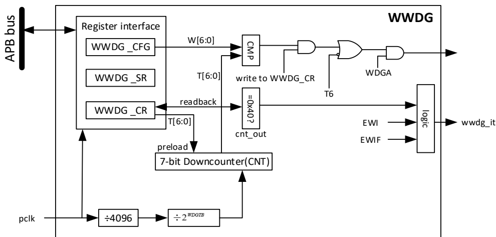
图 20-1 WWDG 模块框图
