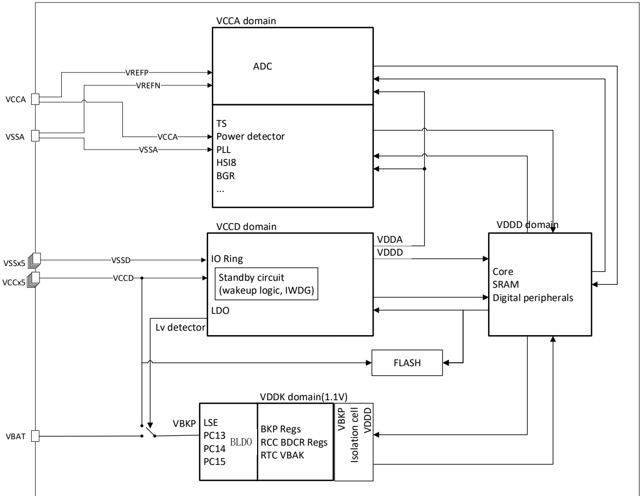
图 4-1 电源结构
