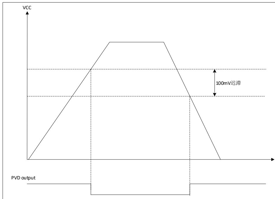
图 4-3 PVD 时序
