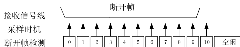
图 27-7 LIN 模式下的断开帧长度不够的情况
