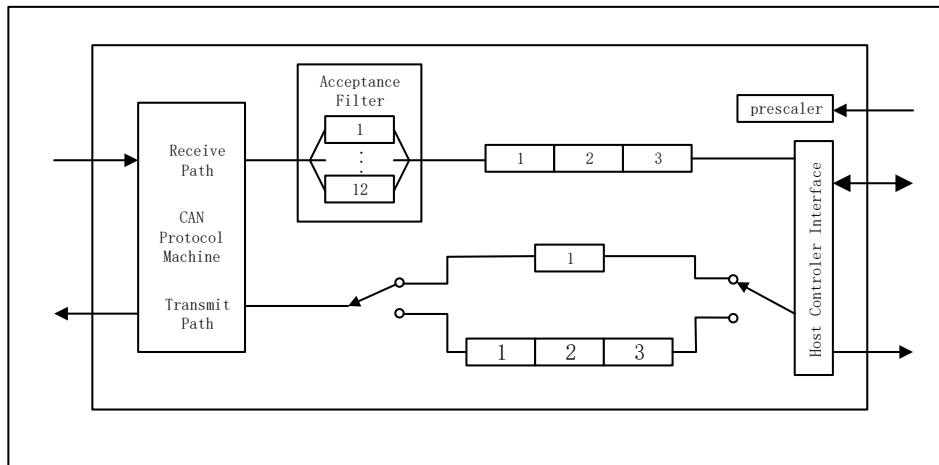
图 24-1 CAN FD 模块框图
